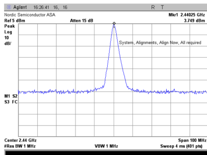
Mid +4dBm Fundamental
