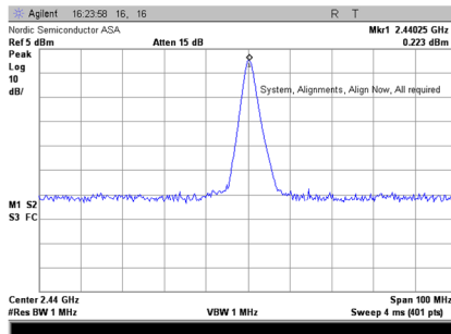
Mid 0dBm Fundamental
